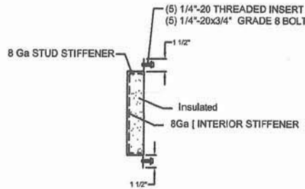
STUD STIFFENER
