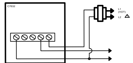
Fig. b Wiring for C7632
