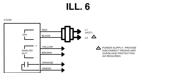
Fig. a Wiring for C7232
